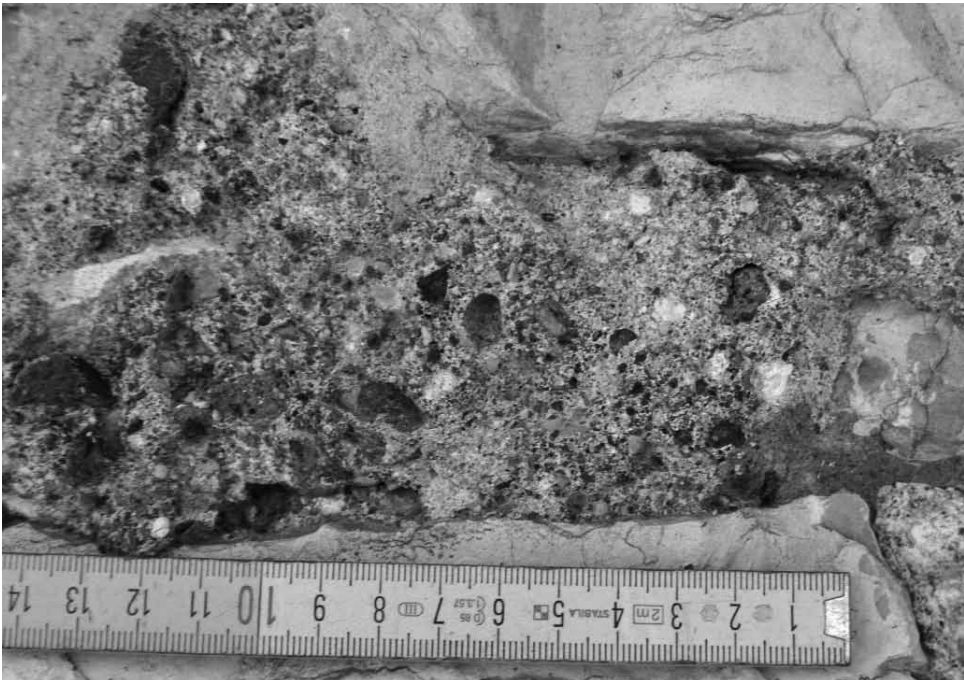
11. Torre di piazza: tecnica muraria del periodo III, particolare metrico della malta di finitura
