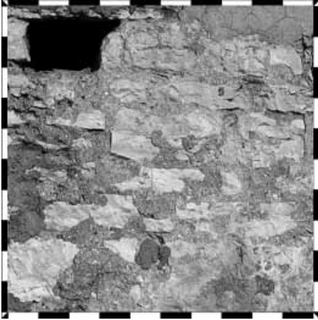
10. Torre di piazza: tecnica muraria del periodo III, campione metrico di muratura sul lato ovest
