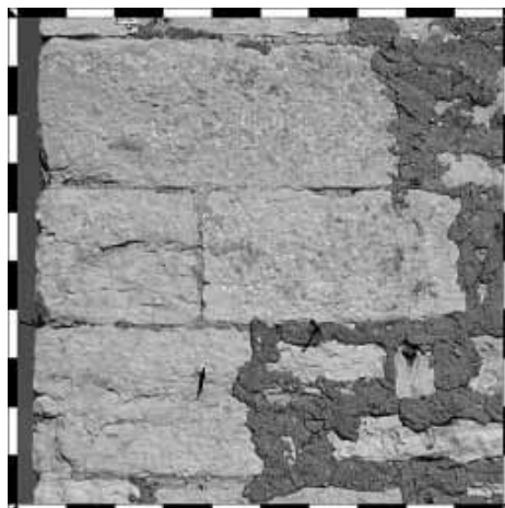
12. Torre di piazza: tecnica muraria del periodo III, campione metrico della muratura in corrispondenza dell'angolata nord-ovest
