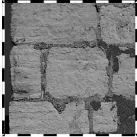
7. Torre di piazza: tecnica muraria del periodo II, campione metrico della muratura in corrispondenza dell'angolata nord-ovest
