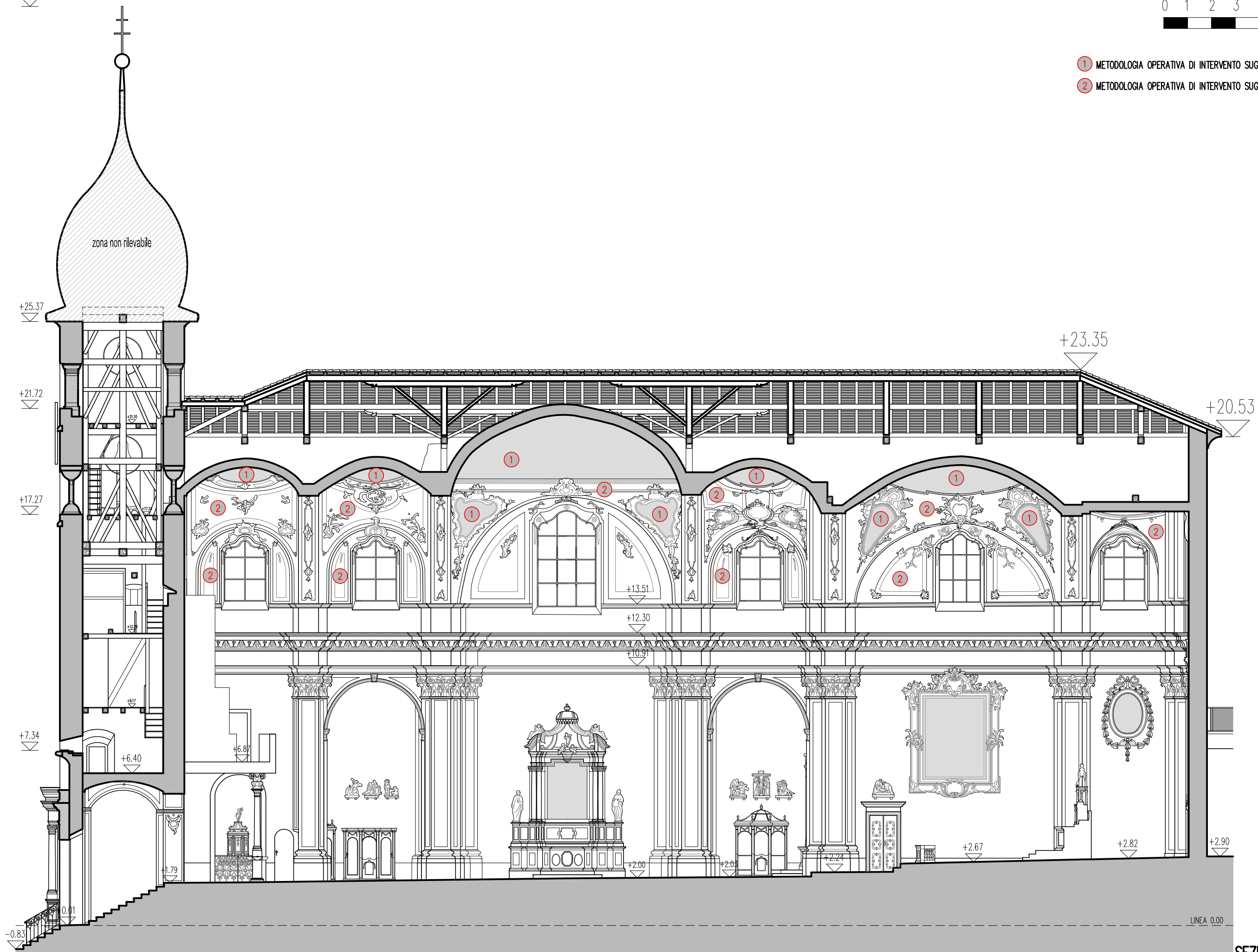
SEZIONE A-A
