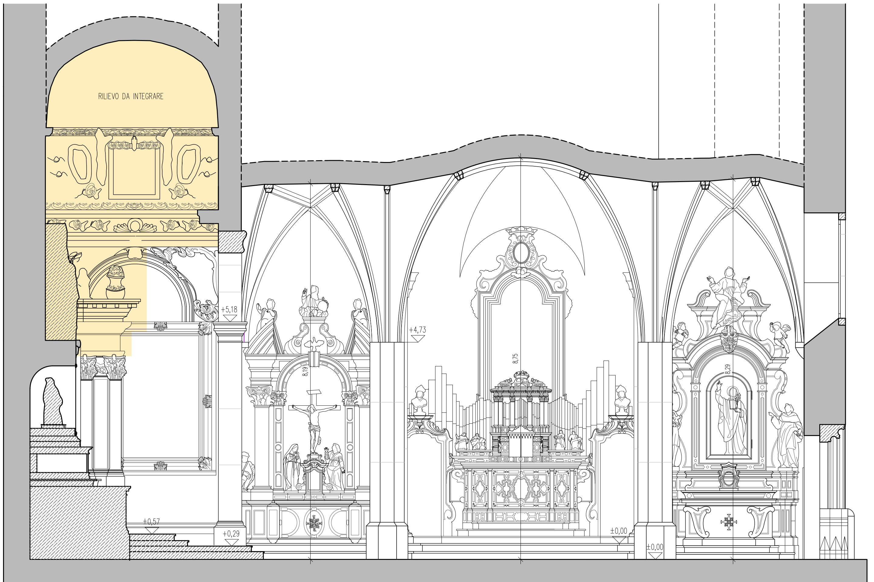
SEZIONE B-B - scala 1:50
